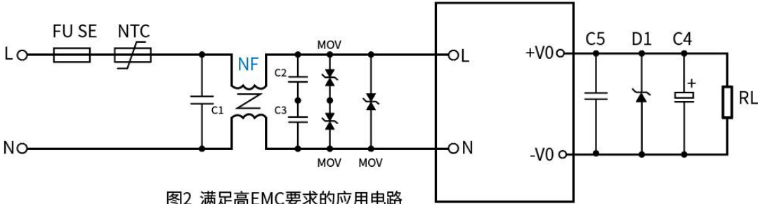
图2 满足高EMC要求的应用电路
